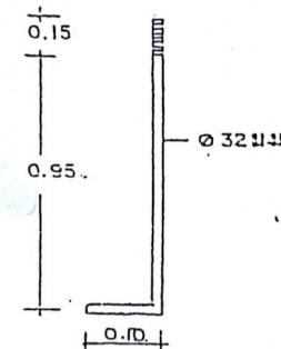
DETAIL ANCHOR BOLT.
