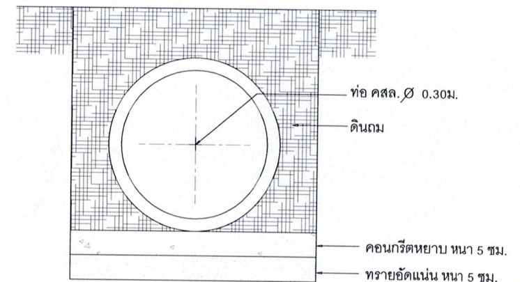
รูปตัดA ท่อ คสล.
