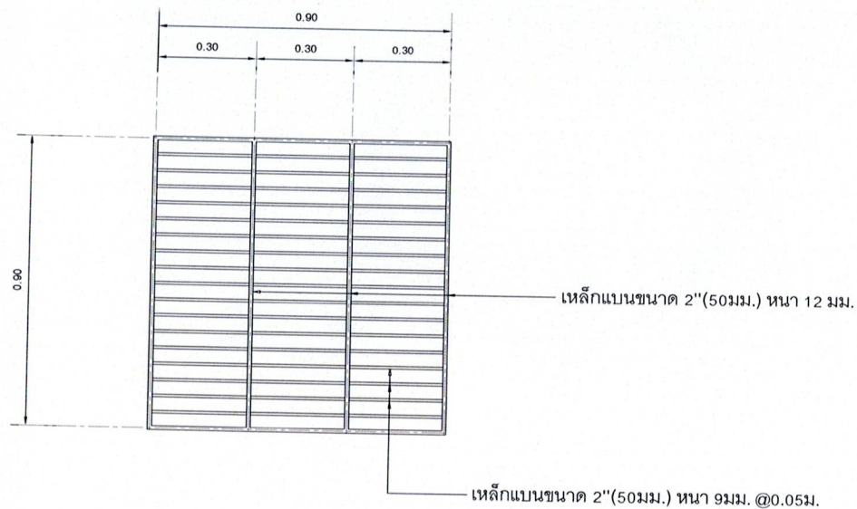
ขยายฝาบ่อพัก
