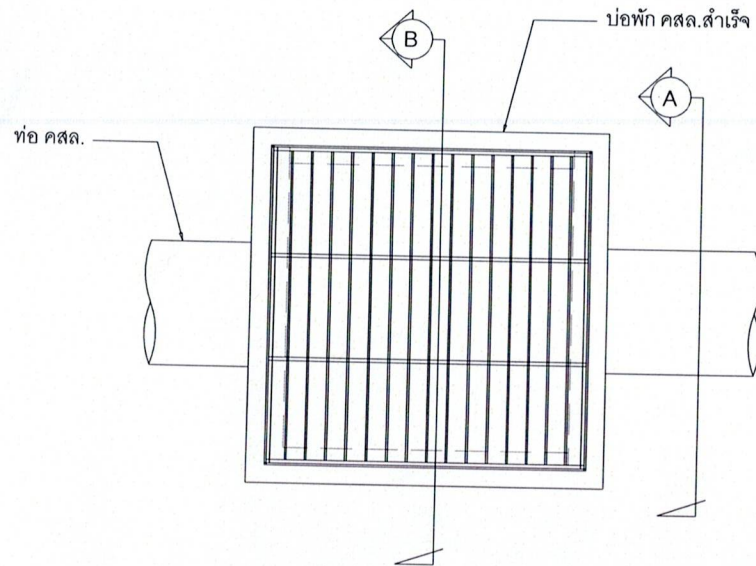
แปลนบ่อพักคอนกรีตสำเร็จรูป
