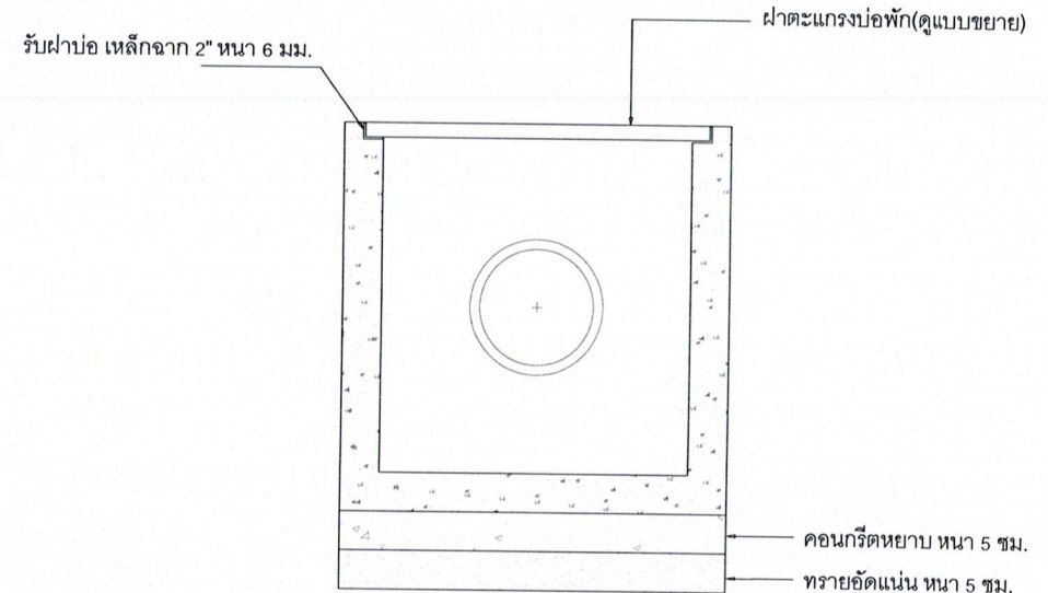
รูปตัดB บ่อพักคสล.สำเร็จรูป
