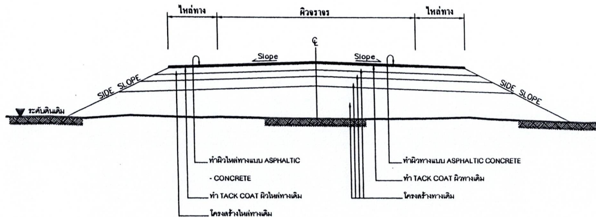
ข้อกำหนดในการเสริมผิวลาดยางแอสฟัลติกคอนกรีต
