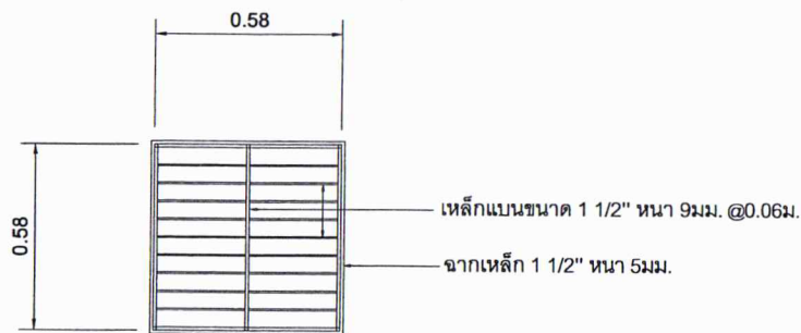
ขยายฝาบ่อพัก
