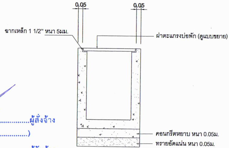
บ่อพักคอนกรีตสำเร็จรูป สำหรับ ท่อ คสล. Ø 0.30ม.
