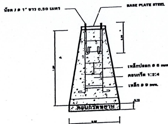
ฐานวางเสาไฟฟ้าถนนกิ่งเดียว
