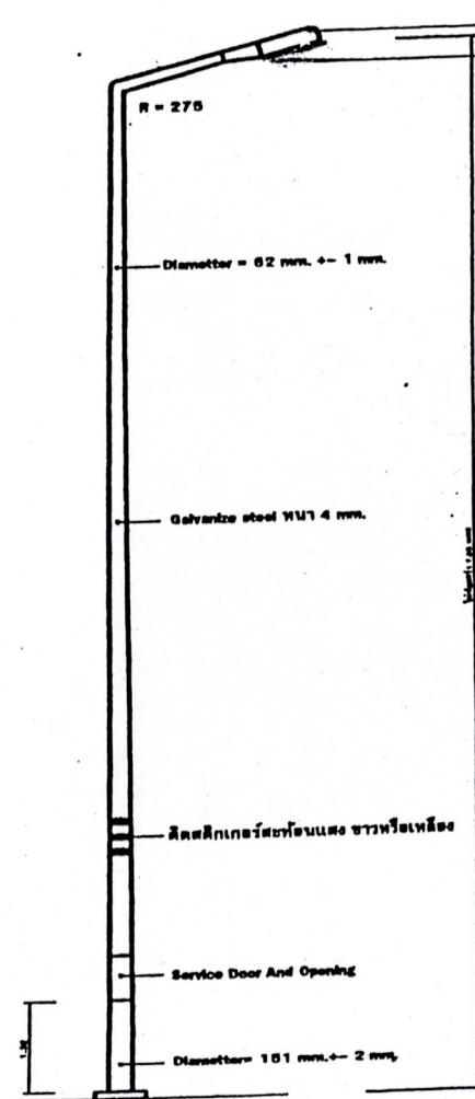
เสาไฟฟ้าถนนกิ่งเดียว
