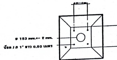
แป้นฐานวางเสาไฟฟ้าถนนกิ่งเดียว
