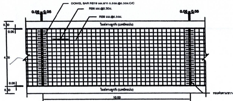
แปลนแสดงการเสริมเหล็กถนน คคค. NOT TO SCALE
