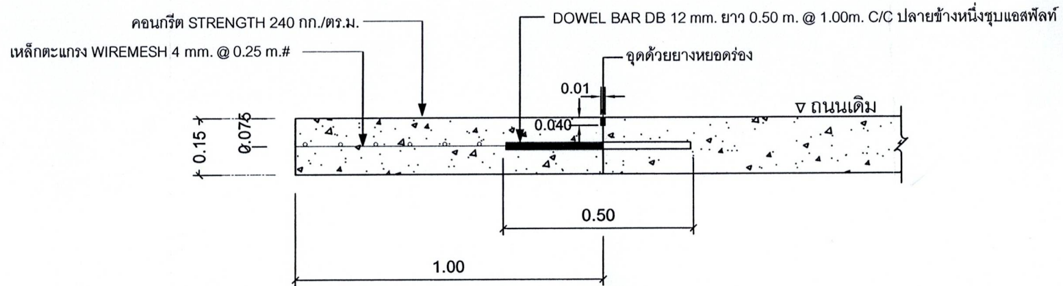
ขยายรอยต่อ CONTRACTION JOINT2
