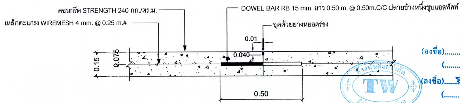
ขยายรอยต่อ CONTRACTION JOINT1
